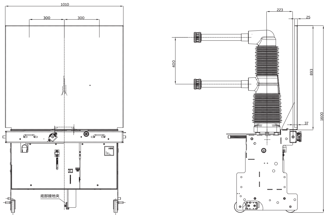
手车式P300大面板外形尺寸
