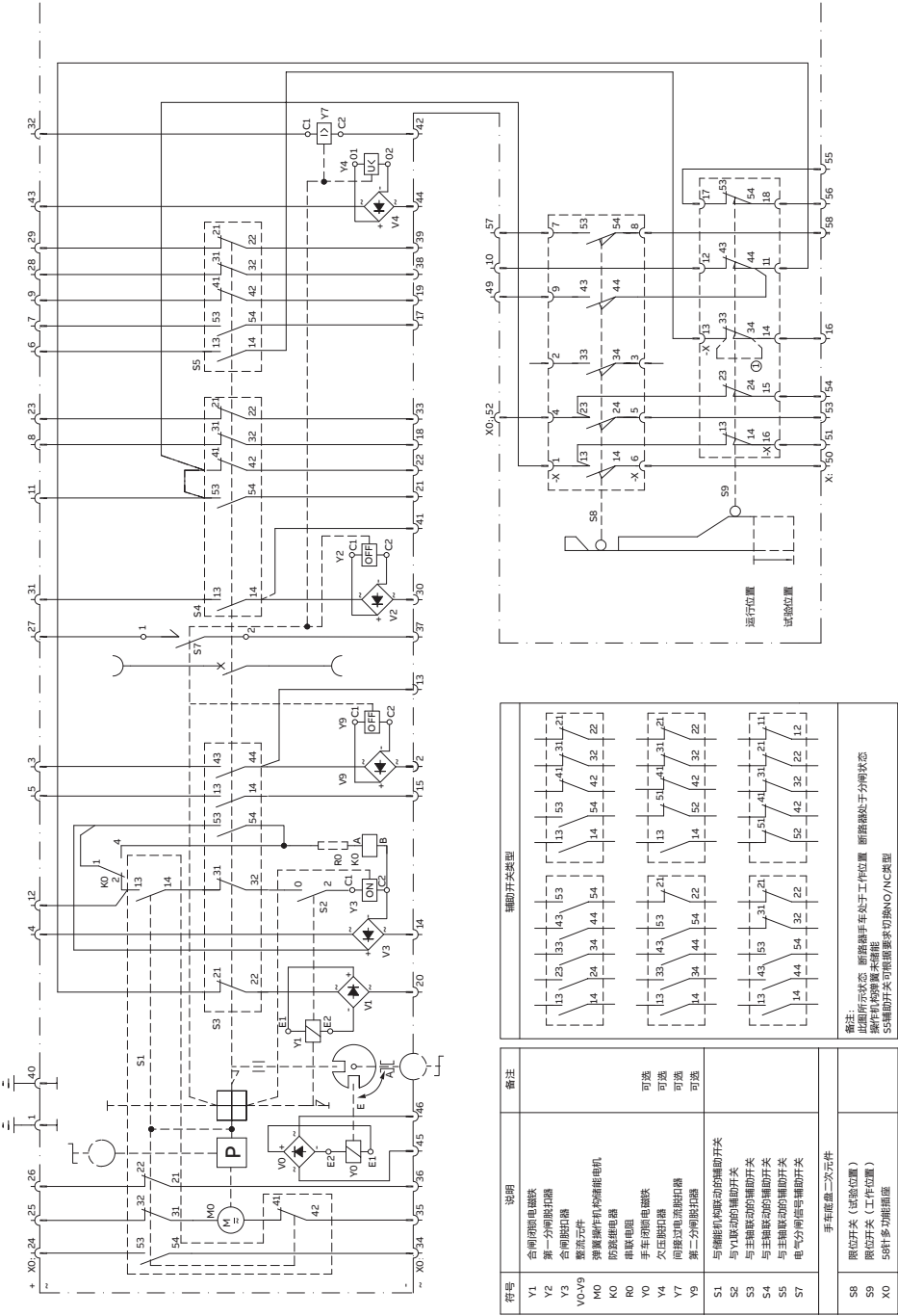
可抽出式5NO-6NC电气图
