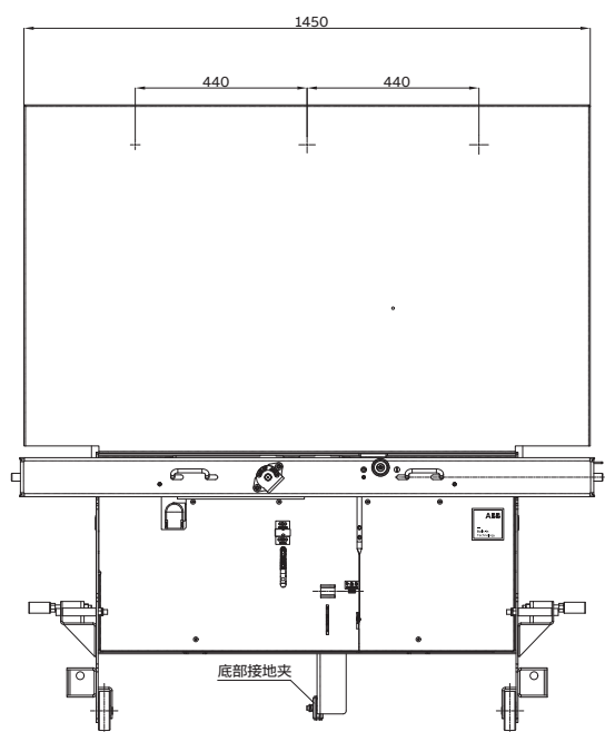
手车式P440大面板外形尺寸
