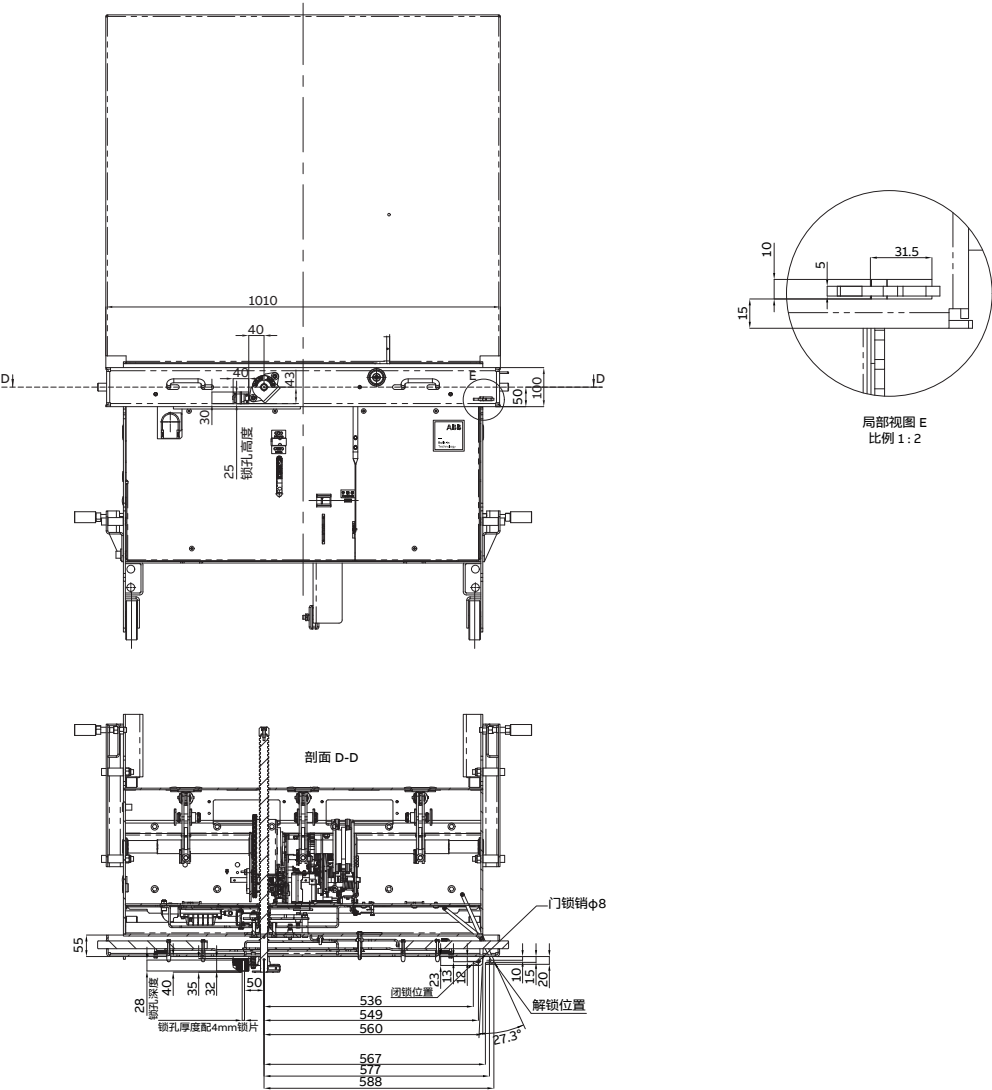
手车式P300关门联锁与柜门闭锁装置（可选配）
